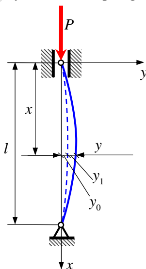
Rys. 7. Wyboczenie pręta o wstępnej krzywiznie
