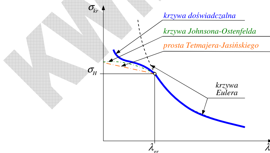
Rys. 6. Zależność naprężeń krytycznych od smukłości pręta ulegającego wybozczeniu Wartość graniczną smukłości wyznacza się z zależności:
