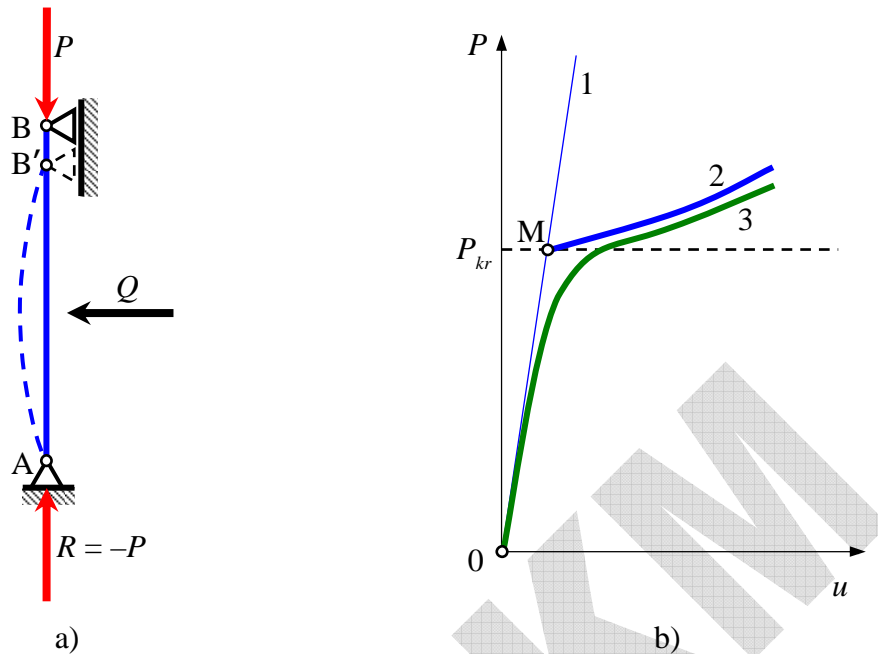
Rys. 3. a) Nieważki pręt ściskany osiowo; b) zależność u - P
